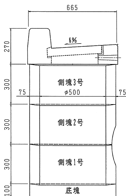
155SF型縁塊組立図
