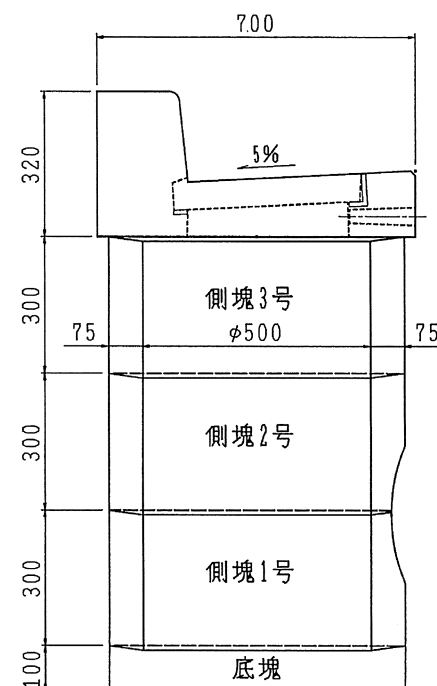
205A・205B型縁塊組立図
