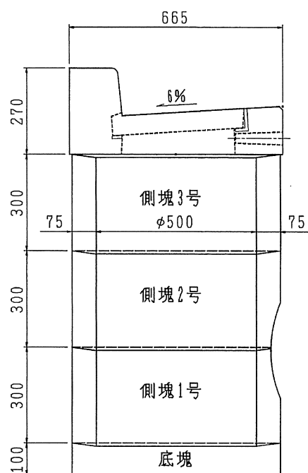
155型縁塊組立図
