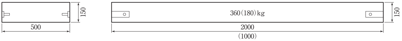
敷設構造図
