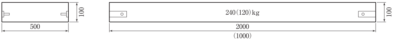
敷設構造図
