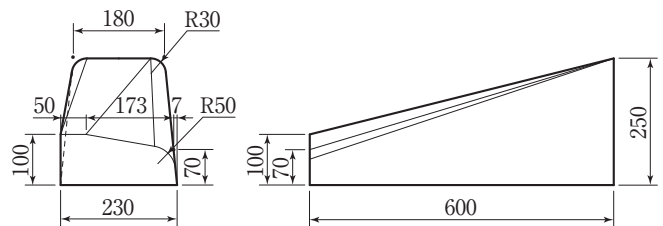
両面歩車道B1本斜Ⅲ型平用
