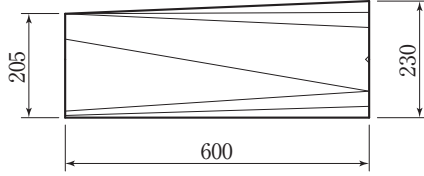
両面歩車道B1本斜SF用
