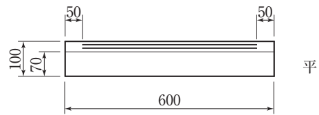
Ⅲ型平ブロック
