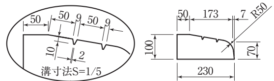
両面歩車道B1本斜Ⅲ型平用
