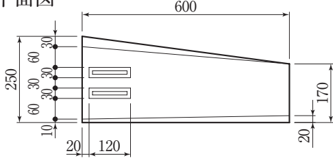
歩車道 A (斜ブロック L=600)
