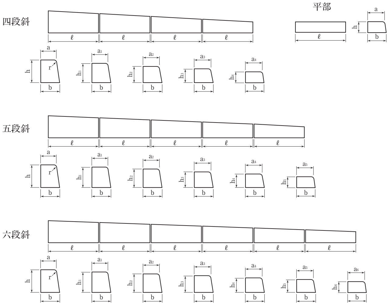
仕様寸法表(単位mm)
