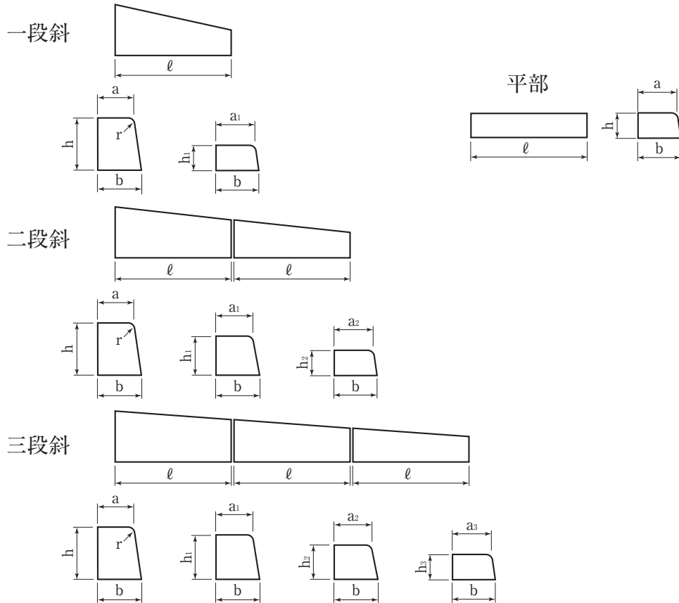
仕様寸法表(単位mm)
