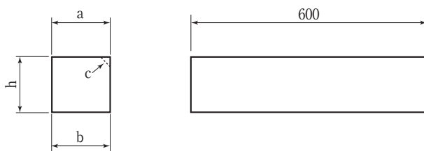
地先境界ブロック
