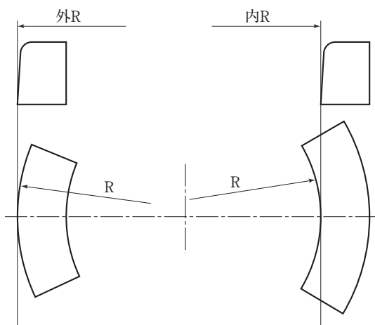
片面歩車道境界ブロック曲り
