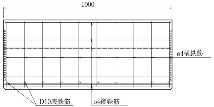
横断用(T-20、25)
